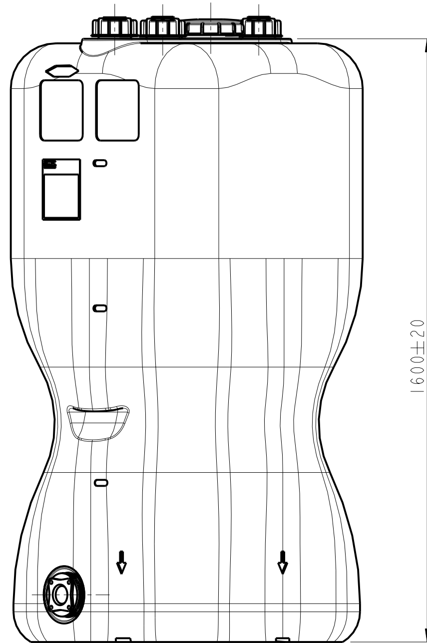
Ansicht A
